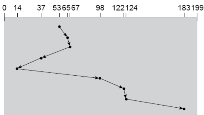
Figura 5. Planificación de disco Shortest-Seek-Time-First [Silberschatz2010].
